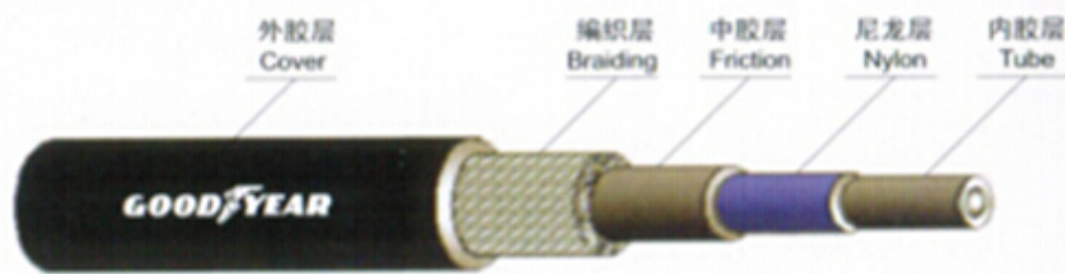
空调管产品结构图 A/C Hose Construction
